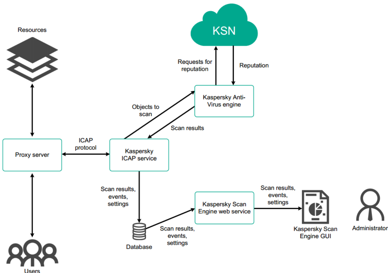
Рисунок 2. Взаимодействие прокси-сервера и Kaspersky Scan Engine в режиме ICAP
